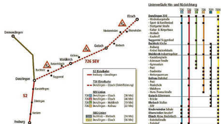
Elektrifizierung Elztalbahn Denzlingen – Elzach 01.03. – 12.12.2020
